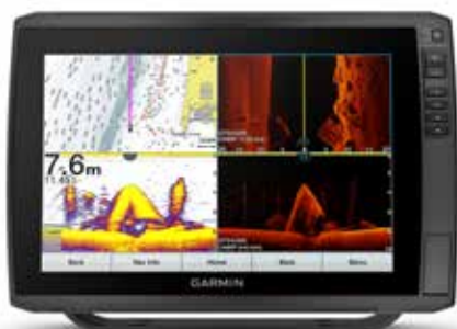
ECHOMAP Ultra 122sv con trasduttore GT56UHD-TM ECHOMAP Ultra 122sv senza trasduttore
